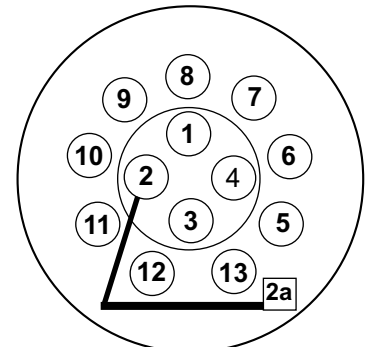
Kontaktbelegung 13 pol der Steckdose
