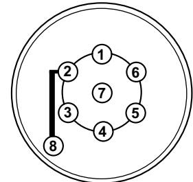
Kontaktbelegung 7 pol der Steckdose
